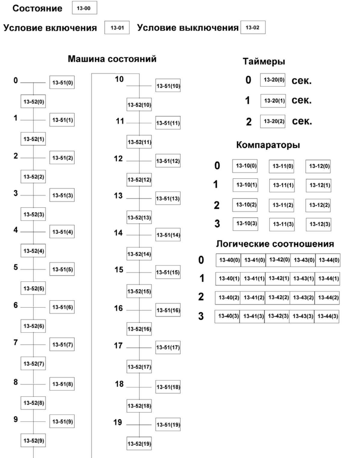
Рисунок 4.21 – Встроенный ПЛК ПЧВ1,2
