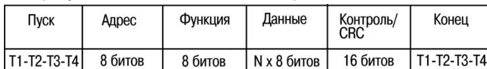
Рисунок 3.2 – Типичная структура сообщения Modbus RTU
